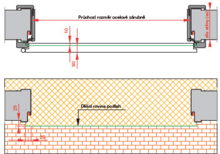
Dveře posuvné na stěnu
